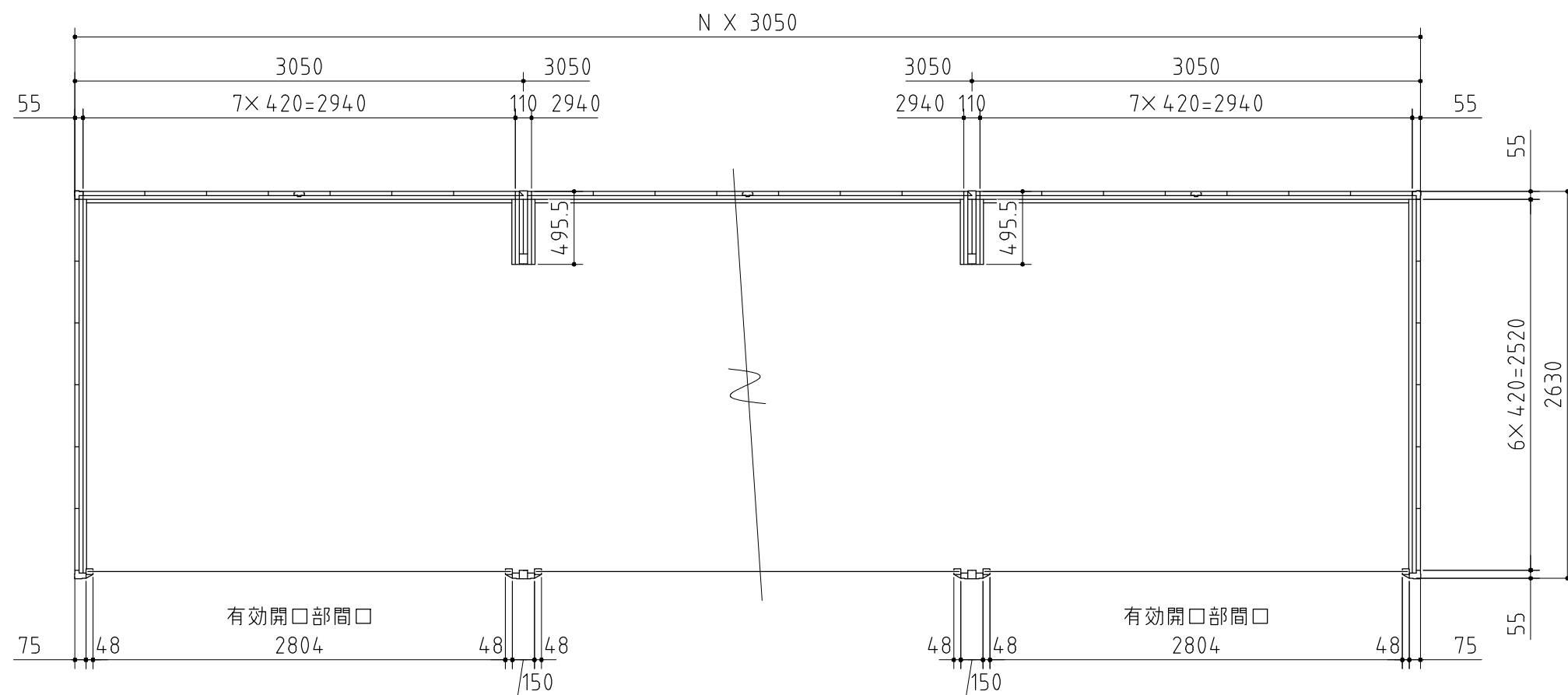
平面図
